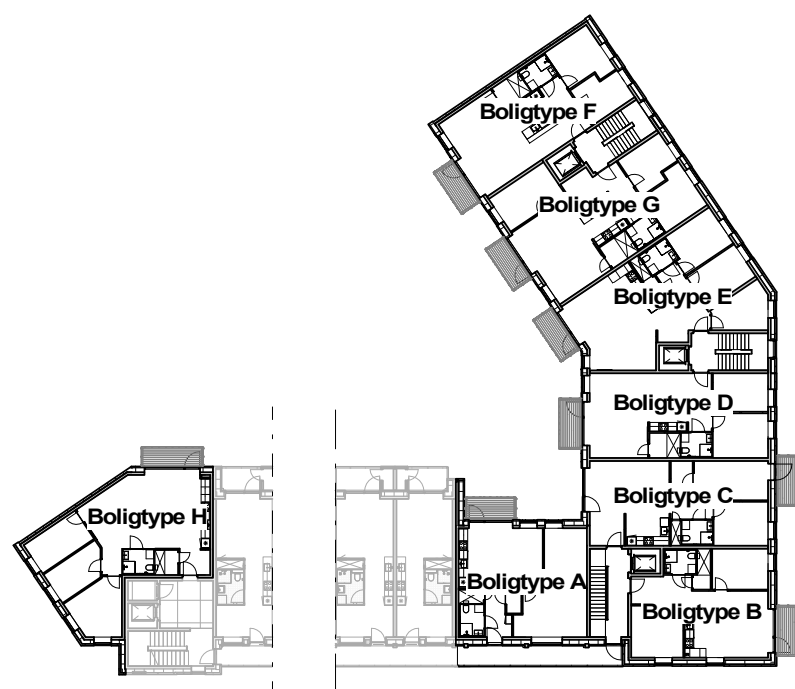
1-5. salsplan
