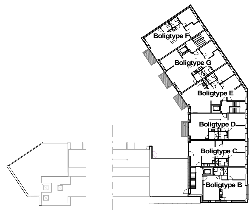
5. salsplan
