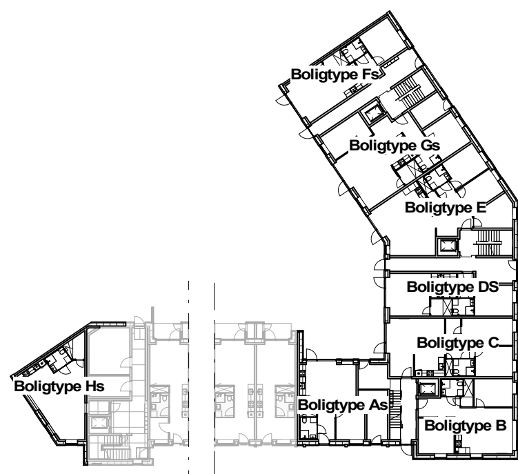
Stueplan
